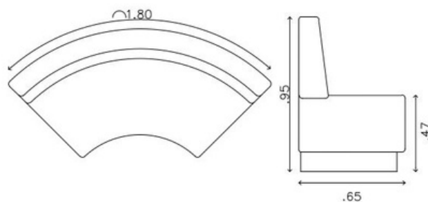
Mínima Curvo (côncavo)
